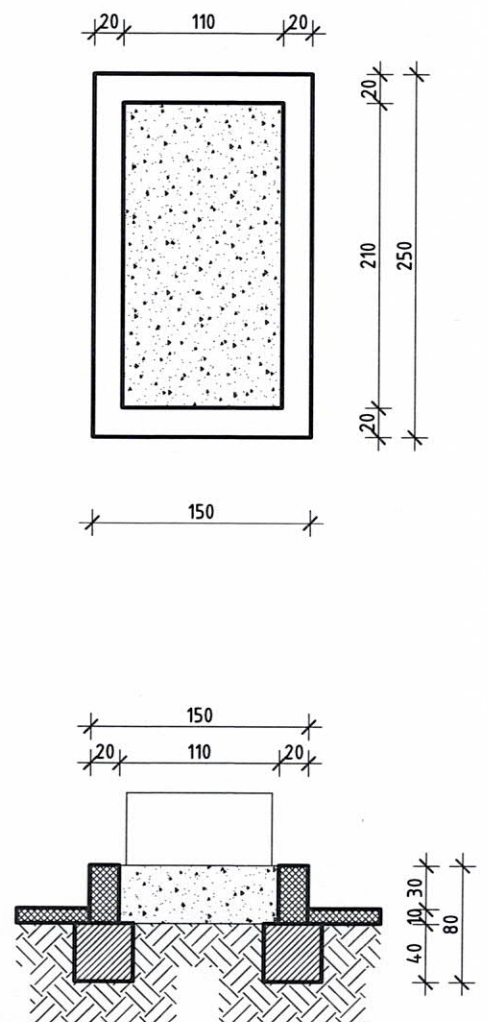
POJEDINAČNO GROBNO MJESTO M 1:50
