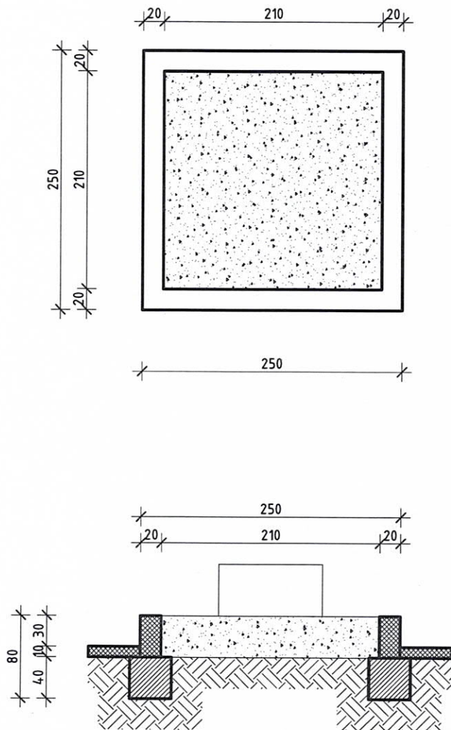
DVOSTRUKO GROBNO MJESTO M 1:50
